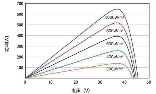
组件的P-V曲线
