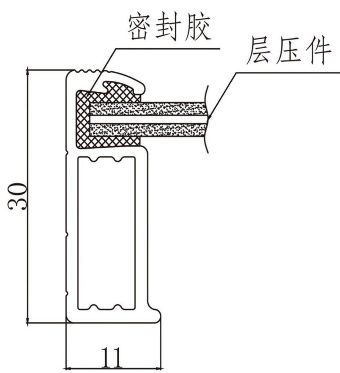
B 短边截面
